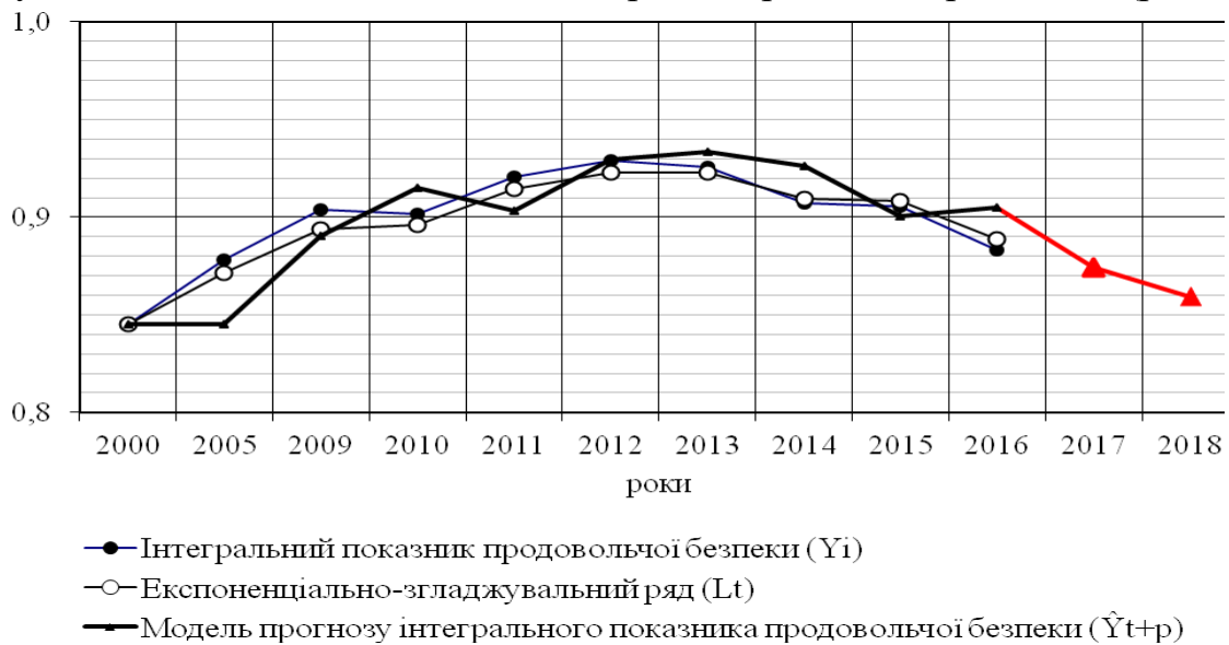
Рис. 8. Модель прогнозу інтегрального показника продовольчої безпеки (розроблено автором)
