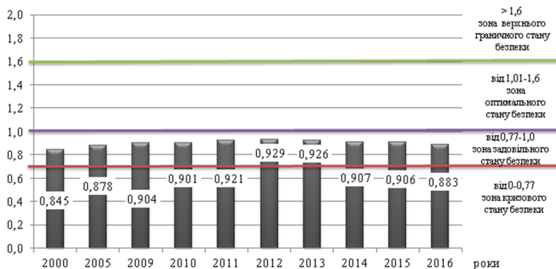
Рис. 7. Стан продовольчої безпеки України за 2000-2016 рр. визначений за допомогою інтегрального показника продовольчої безпеки (розроблено автором)
